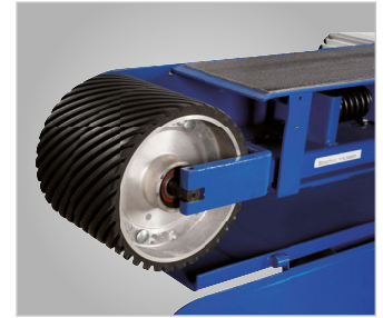
► Velké kontaktní a hnací kolo (obr. MBSM 150-200-2)
