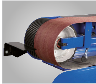
► Rychlá výměna brusného pásu (obr. MBSM 150-200-2)
