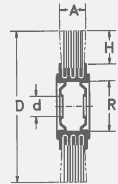
Satynýrovací kartáče
