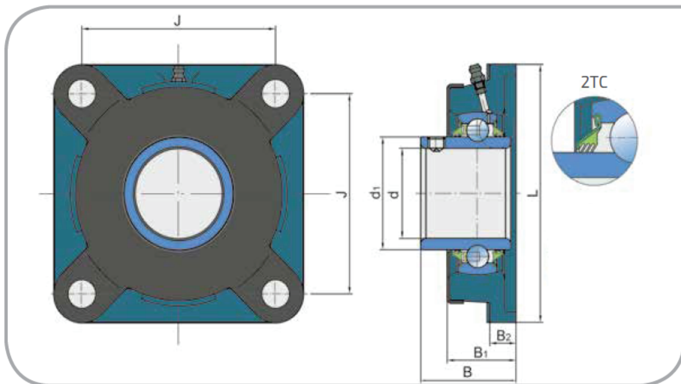
Rozměry/Dimensions (mm)
